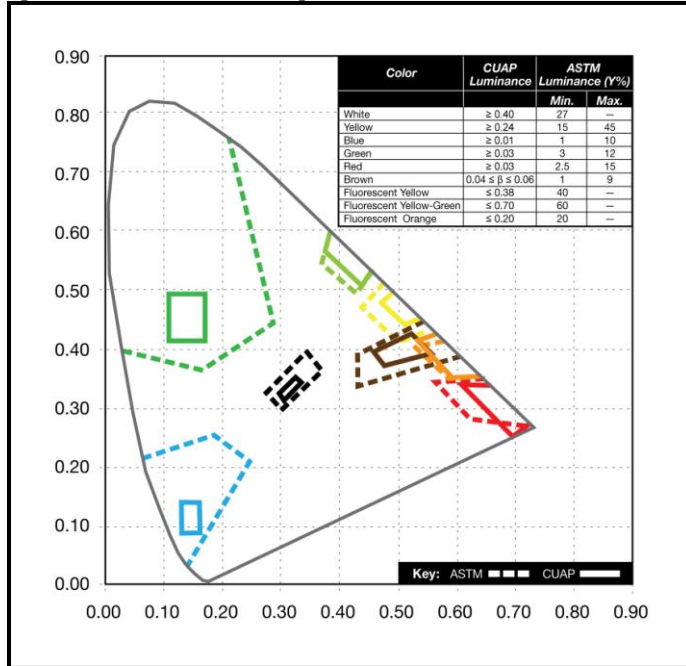
Figura A: Colore diurno – Diagramma CIE dei colori
